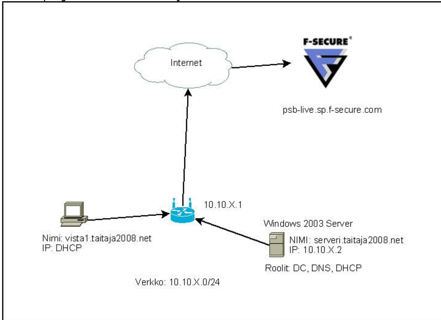
Liite: Topologiakuva Windows Palvelin ja Vista
